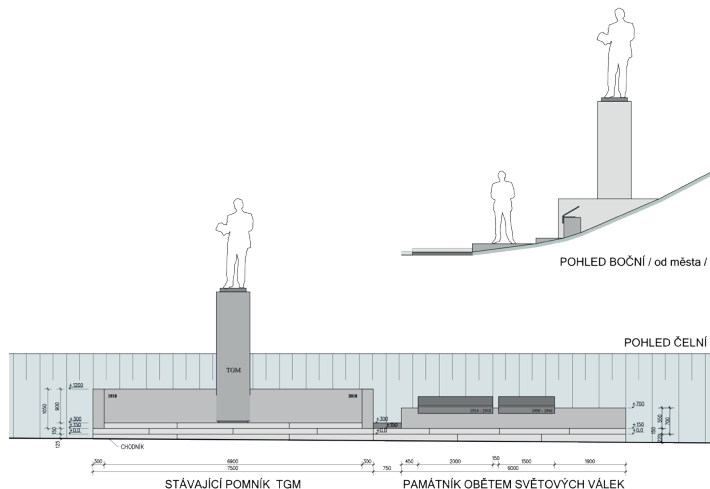
Úprava pomníku TGM a památník obětem světových válek / 1:50
