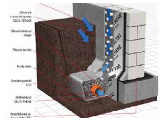
Schéma izolace a drenáže základů.
