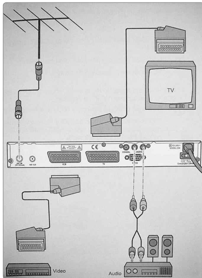
Blokové schéma běžného propojení.
